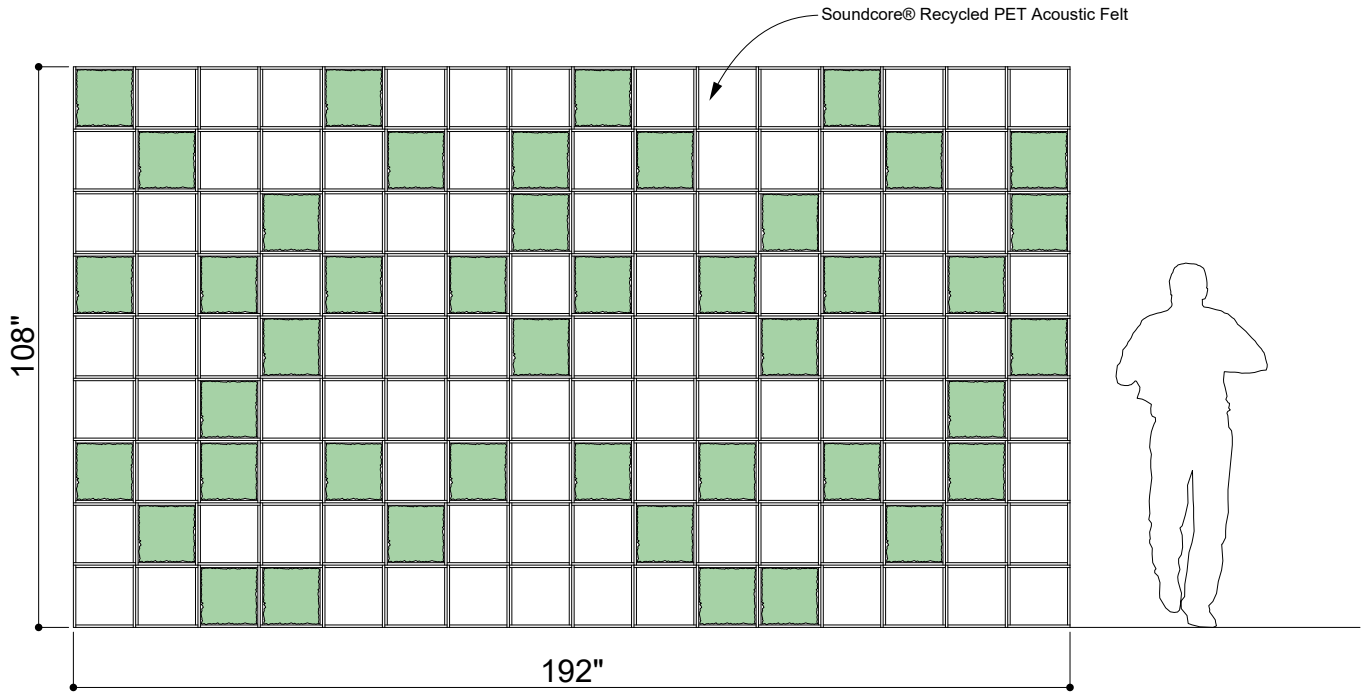
① ELEVATION 1
