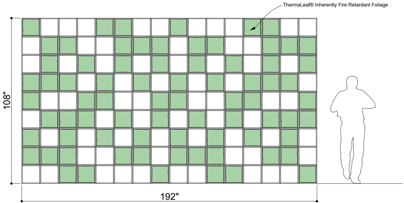
① ELEVATION 2
